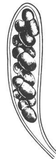
Sporezakje met 8 ascosporen
